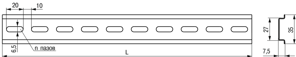
Рисунок 1 – DIN-рейка. Общий вид
